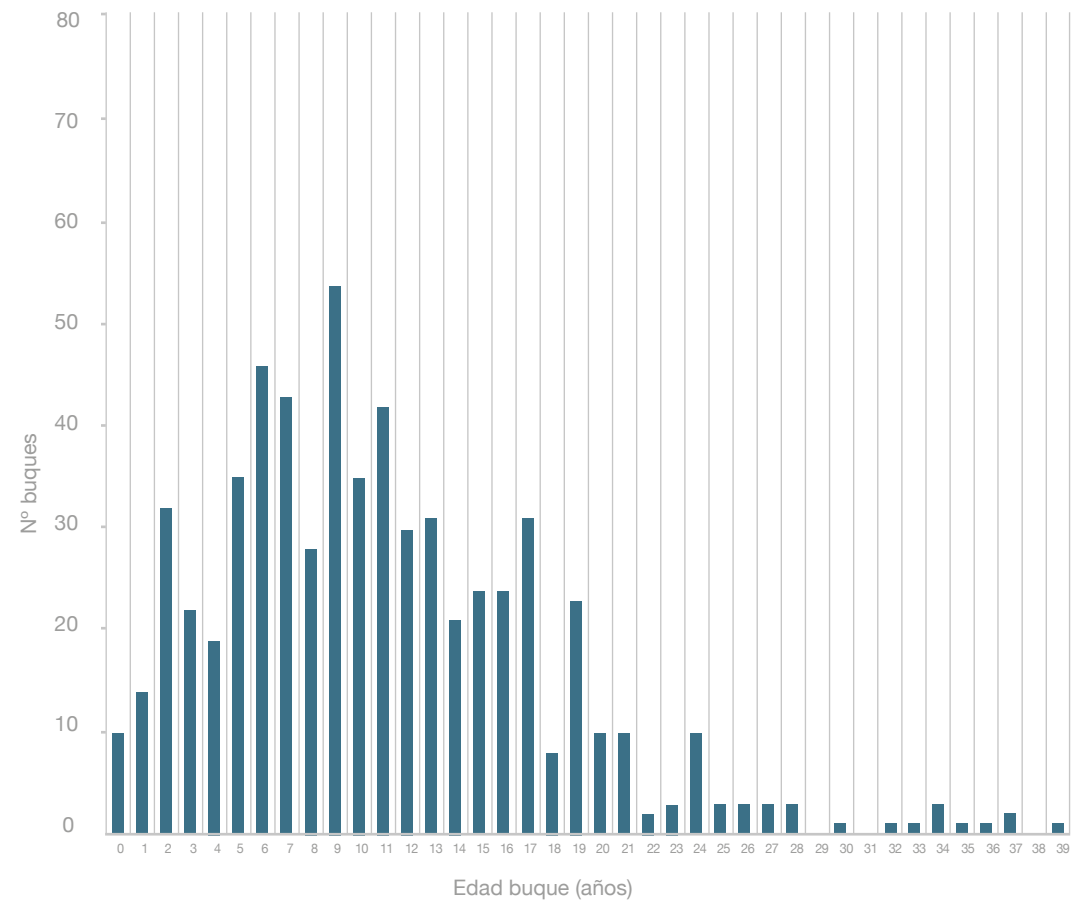
Figura 9. Número de buques según edad
